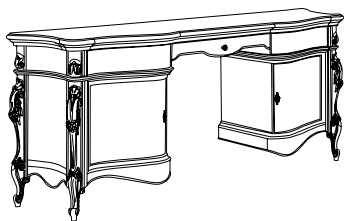
0230F Toilette frassino L. 178 P. 53 H. 78 Peso kg 55 - mc 0,80
