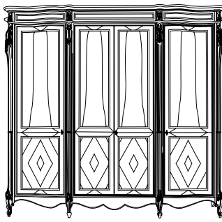
0226N Armadio 4 porte noce L. 296 P. 71 H. 254 Peso kg 250 - mc 3,45
