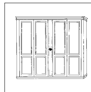
Art. M53 Armadio 4 porte dritte legno (comprensivo cassettiera 6 c.) cm L.305 P.65 H.255 M³ smontati 1,89 M³ montati 5,05 Peso Kg 84 PAG. 28/29
