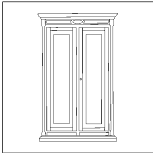
Art. M72 Armadietto 2 porte con segreto cm L.125 P.45 H.202 M³ smontati 0,42 M³ montati 1,14 Peso Kg 42 PAG. 15
