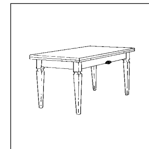
Art. M57 Tavolo rettangolare allungabile con 2 allunghe da 50 cm chiuso cm L.180 P.90 H.80 aperto cm L.280 P.90 H.80 M³ smontati 0,28-M³ montati 1,31 peso Kg 63 PAG. 4/5
