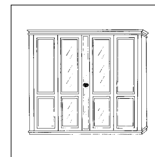
Art. M53/A Armadio 4 porte dritte specchio (comprensivo cassettiera 6 c.) cm L.305 P.65 H.255 M³ smontati 1,89 M³ montati 5,05 Peso Kg 84 PAG. 30/31
