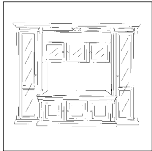
Art. M73/A Componibile (a schema fisso) cm L.290 P.54 H.234 M³ smontati 2,08 M³ montati 3,66 Peso Kg 86 PAG. 22/23
