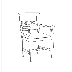
Art. M76 Poltrona rosa cm L. 45,5 P. 52,5 H. 94,5 H. seduta 40,5 Peso Kg 7 PAG. 18
