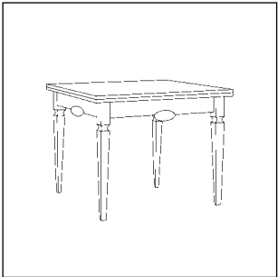
Art. M66 Tavolo quadrato a libro chiuso cm L.100 P.100 H.80 aperto cm L.200 P.100 H.80 M³ smontati 0,18 M³ montati 0,81 Peso Kg 22 PAG. 8/9
