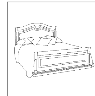
Art. M63 Letto sagomato cm L.175 P.213 H.130 (misura interna cm L.165 P.200) M³ smontati 0,35 M³ montati 4,84 Peso Kg 25 PAG. 32/33
