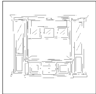
Art. M73 Componibile con cassetti (a schema fisso) cm L.290 P.54 H.234 M³ smontati 2,08 M³ montati 3,66 Peso Kg 92 PAG. 24/25
