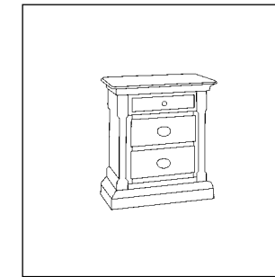
Art. M50 Comodino 3 cassetti cm L.53 P.38 H.64 M³ 0,13 Peso Kg 18 PAG. 32
