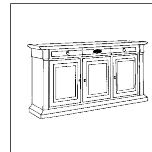
Art. M60 Credenza 3 porte + 3 cassetti cm L.206 P.55 H.106 M³ 1,21 Peso Kg 62 PAG. 6
